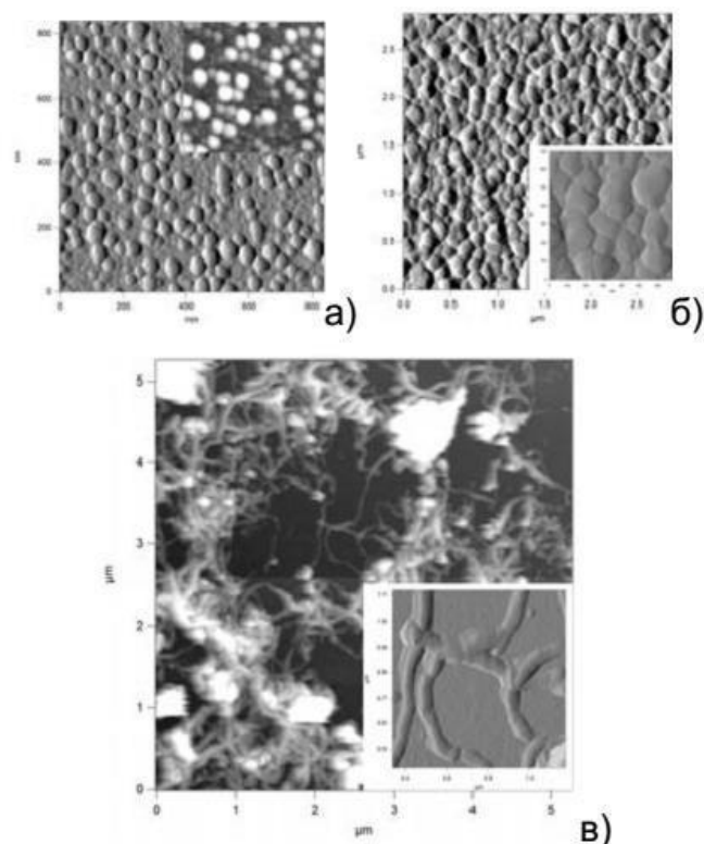
Рисунок 3. – АСМ-изображение поверхности гетероконтактных систем TiO 2 -Полиимид
