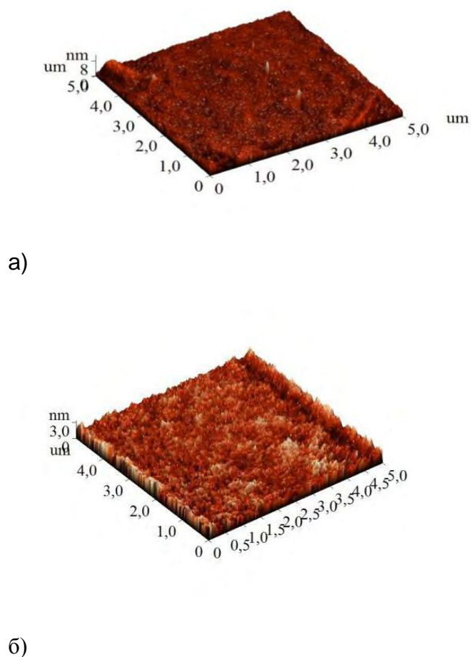
Рисунок 1. – АСМ-изображение пленок а) TiO 2 (0,5 вес.%), б) TiO 2 (0,05 вес.%)
