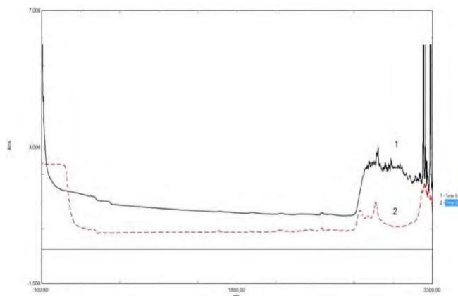
Рисунок 2. – Спектры поглощения пленок TiO 2 – Полиимид (1 – 0,5 вес.%, 2- 0,05 вес.%)
