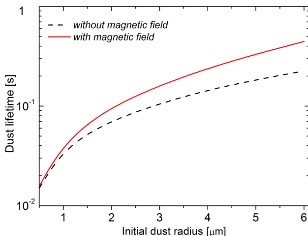
Рисунок 4 - Время жизни пылинки в однородной дейтериевой плазме в присутствии (сплошная линия) и без учета (пунктирная) магнитного поля в зависимости от радиуса пылинки
