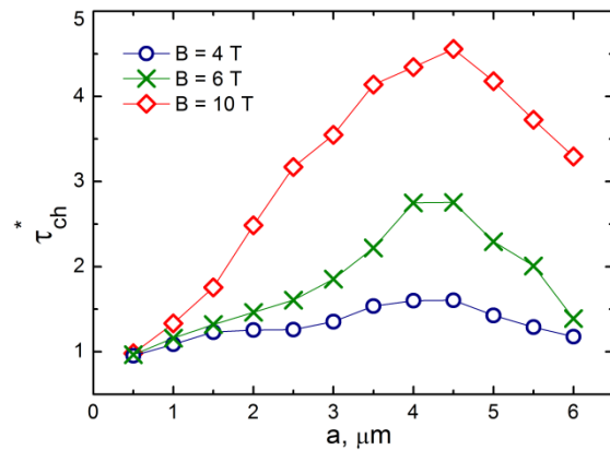
Рисунок 3 – Отношение времени зарядки пылевых частиц в присутствии/без учета магнитного поля в зависимости от радиуса пылинки
