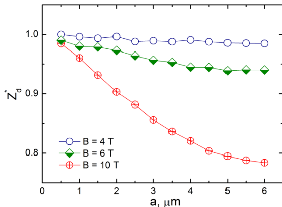
Рисунок 2 - Отношение заряда пылевых частиц в присутствии/без учета магнитного поля в зависимости от радиуса пылинки
