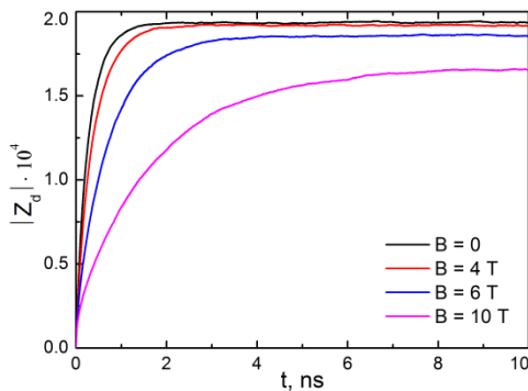
Рисунок 1 – Временное распределение заряда пылевой частицы ( a=3\mu\text{m} ) при различных значениях магнитного поля
