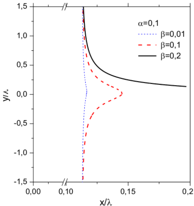
Рисунок 4 – Траектория пылинки на пылинке при различных значениях безразмерного параметра \beta
