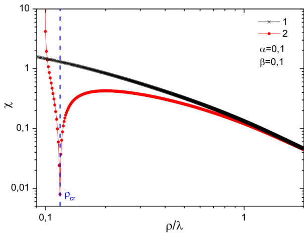
Рисунок 3 - Угол рассеяния в зависимости от нормированного прицельного параметра \rho/\lambda
