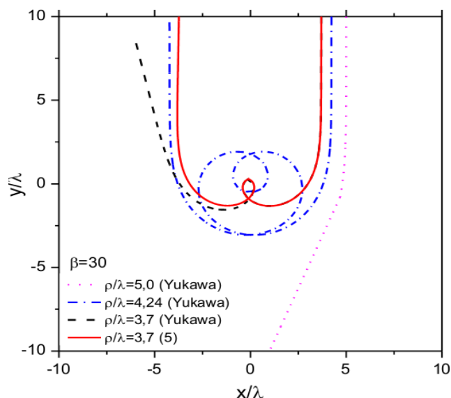
Рисунок 2 – Траектория иона на пылинке при различных значениях прицельного параметра \rho / \lambda ( \rho_* \cong 4.24\lambda )
